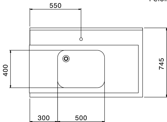
Felülnézet
